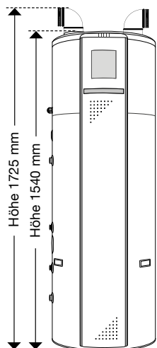
Ø 650 mm Kippmass: 165 cm
