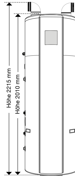
Ø 750 mm Kippmass: 212 cm
