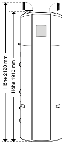
Ø 750 mm Kippmass: 202 cm
