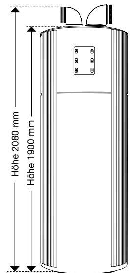
Ø 650 mm Kippmass: 200 cm
