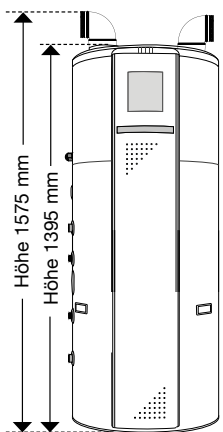
Ø 650 mm Kippmass: 152 cm
