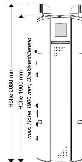
Ø 650 mm Kippmass: 200 cm
